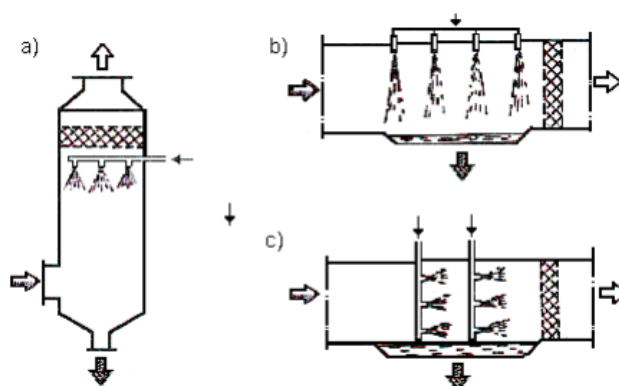
Figura 1 - Configurações possíveis de lavadores de gases: a) contra corrente b) cruzado e c) concorrente, em relação ao fluxo de gás.
