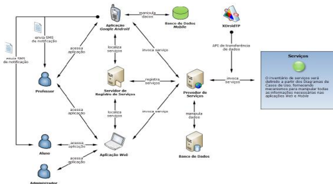
Figura 1 - Modelo da arquitetura do ambiente distribuído.
