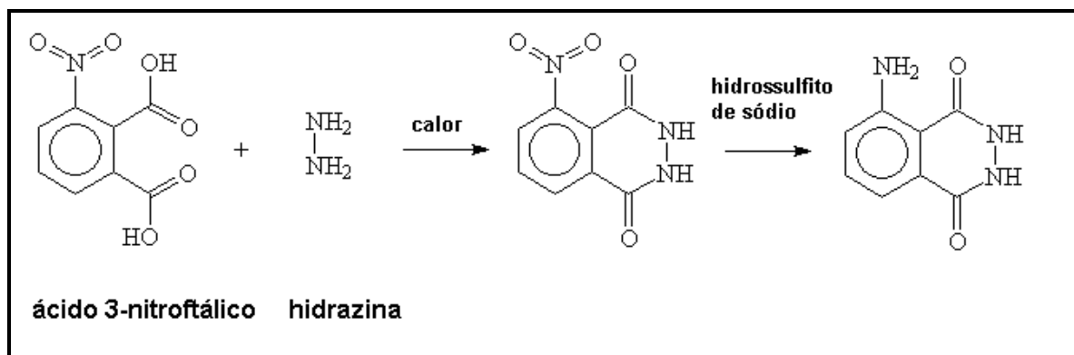
Figura 2: Esquema da síntese do luminol
