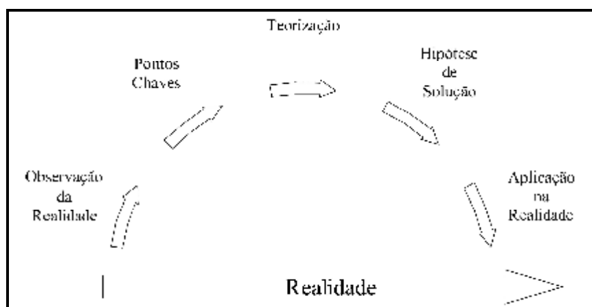
Figura 1 – Teoria do Arco de Maguerz.
