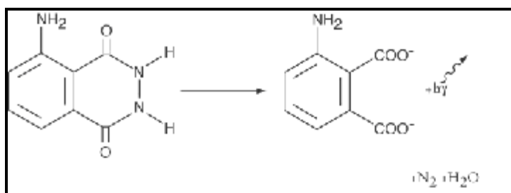
Figura 1: Reação de oxidação do luminol
